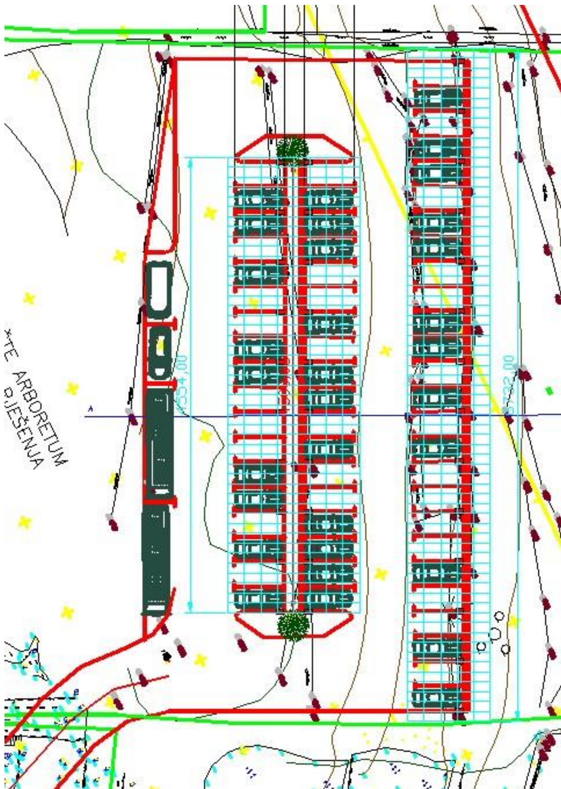
Izvadak iz glavnog projekta uređenja internog parkirališta – tlocrt.
